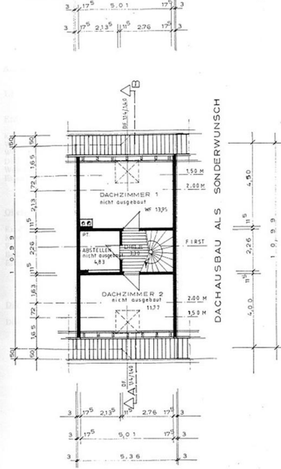
DACHGESCHOSS M. 1 : 1 0 0
