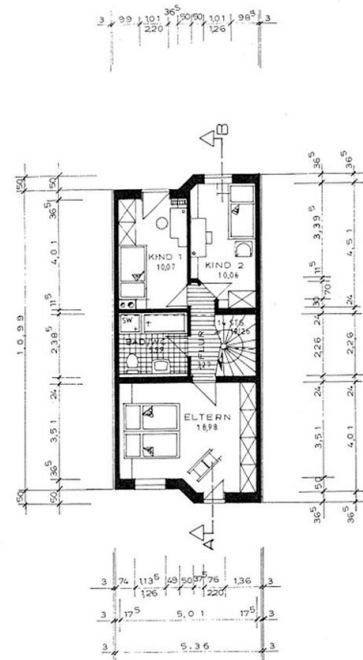
OBERGESCHOSS M. 1 : 1 0 0
