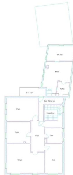
Obergeschoss 1 100
